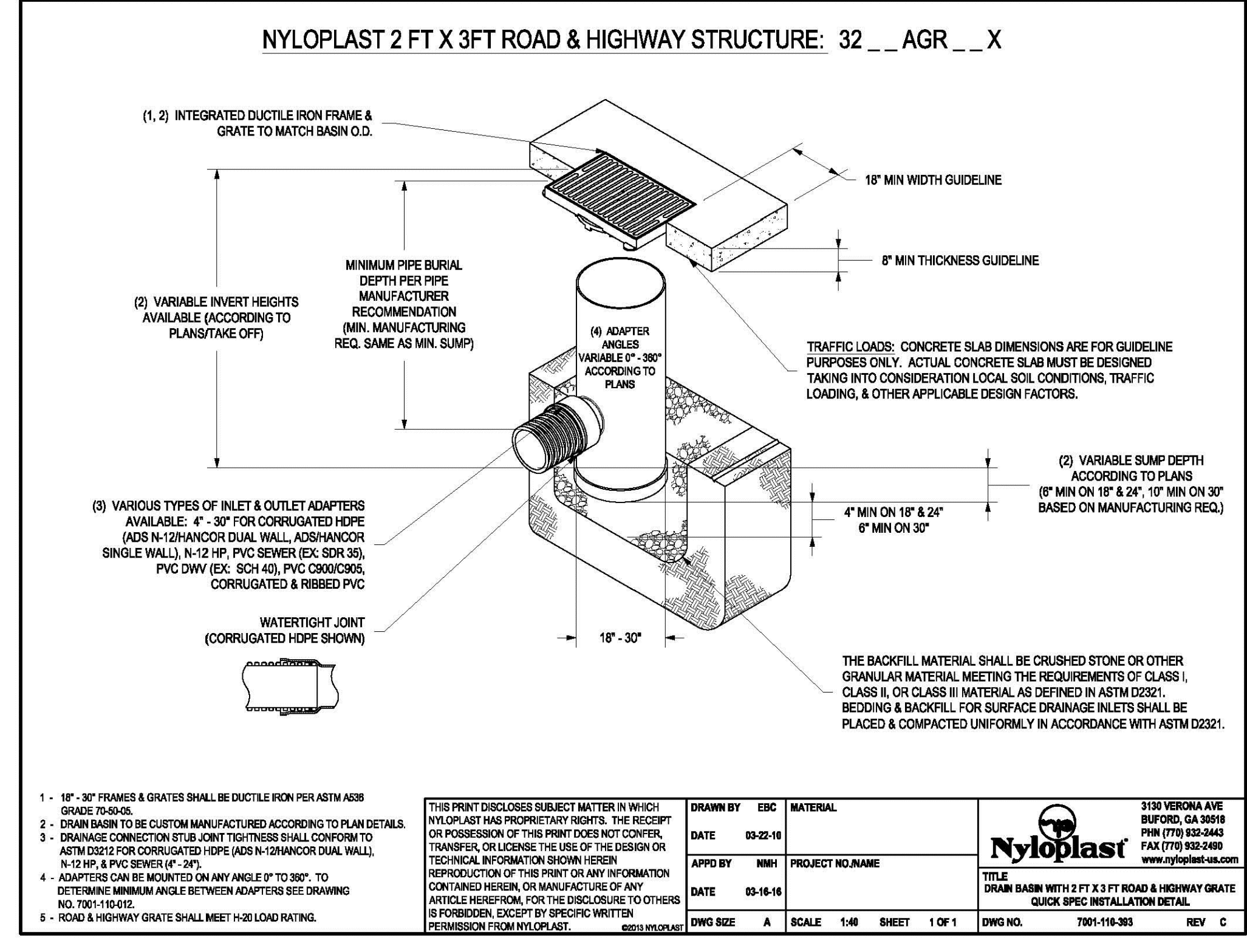
11 NYLOPLAST STRUCTURE N.T.S.
